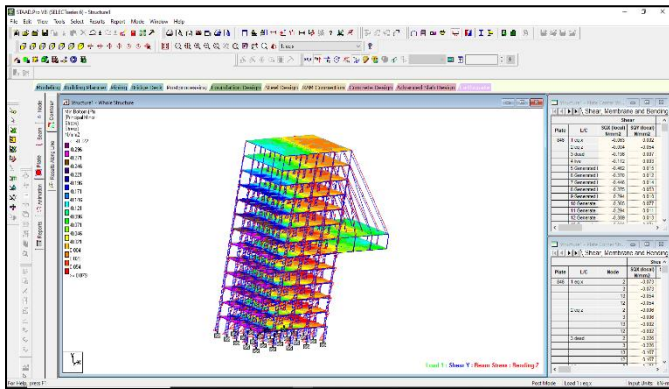
(D) Stress Analysis –Bending Moment.
