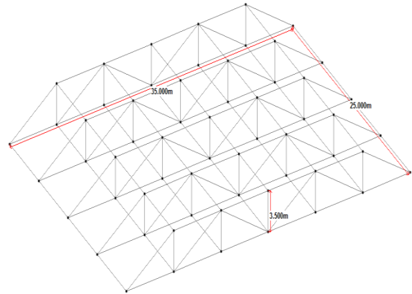
Fig 2 : Howe truss
