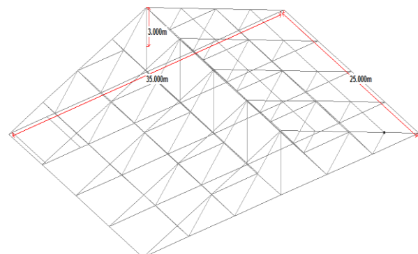
Fig 4 : Flink Truss
