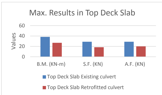
Fig: 11 Top Deck Slab
