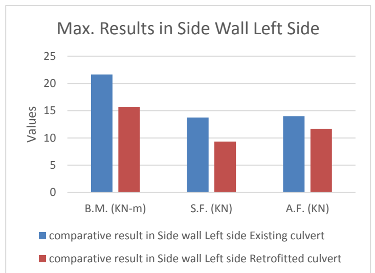
Fig,9 Left hand side wall
